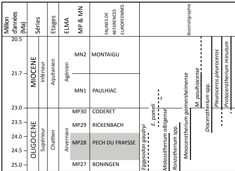
Fig. 4: Biostratigraphie des Rhinocerotidae de l'Oligocène européen, en accord avec les faunes de référence européennes (en capitale). Les corrélations chronologiques et stratigraphiques sont d'après Berger (2011). Les occurrences biostratigraphiques des taxons de Rhinocerotidae sont d'après Uhlig (1999), Antoine et al. (2011), Antoine & Becker (2013) et Scherler et al. (2013). ELMA ( European land mammal ages ): âges basés sur des assemblages de mammifères continentaux européens. Zone grise: âge de la localité d'Éclépens.
