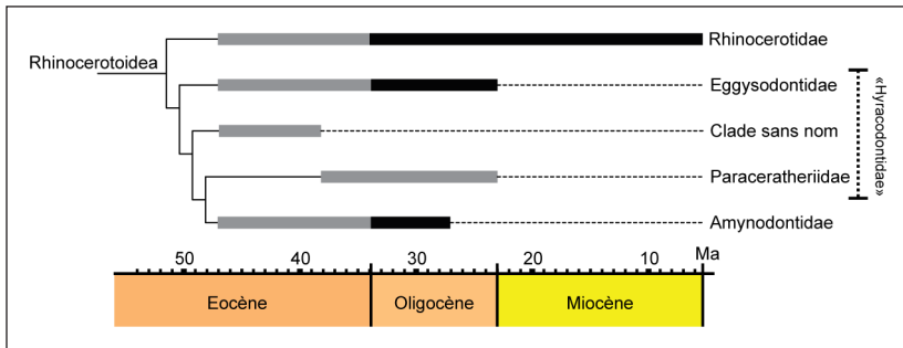
Fig. 1: Arbre phylogénétique simplifié des Rhinoceroidea (modifié d'après Tissier et al. 2017). Les occurrences des différents groupes sont indiquées par des barres grises. Les barres noires correspondent aux occurrences en Europe occidentale.
