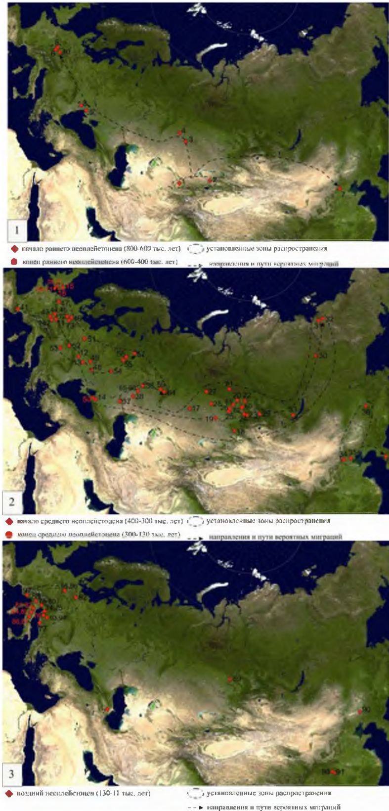
Рис. 1. Карты предполагаемого распространения и расселения Stephanorhinus kirchbergensis в пределах Северной Евразии на основе местонахождений остатков раннего – позднего неоплейстоцена: 1 – ранний неоплейстоцен, 2 – средний неоплейстоцен, 3 – поздний неоплейстоцен. Номера местонахождений соответствуют номерам в таблице
