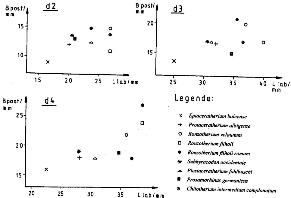
Abb. 3: Längen-Breiten-Diagramme der unteren Milchmolaren von Epiaceratherium bolcense und einigen Vergleichsarten
