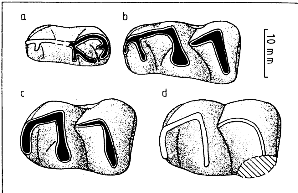
Abb. 2: Untere Milchmolaren und m1 von Epiaceratherium bolcense ABEL 1910, Monteviale (Italien), Unteroligozän, Museo di Geologia e Paleontologia dell'Università di Padova, Nr. 28011. – a: d2; b: d3; c: d4; d: m1; alle dext. und occlusal
