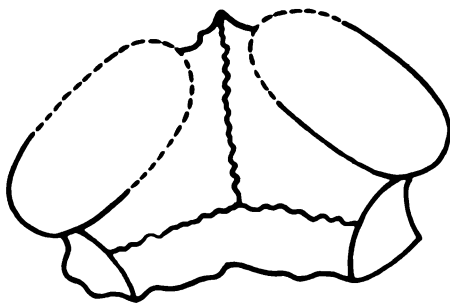
Рис.5. Сечение рогов фронетрагуса
