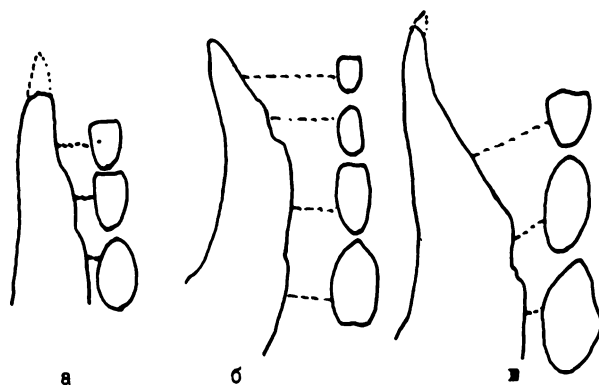
Рис.6. Схематическое изображение рогов мирибилоцерусов а — аркнетского, б — эльдарского, в — базалетского
