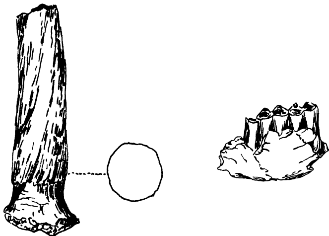
Рис.2. Гипсодонтус из Беломечётской (по Л.К.Габуния, 1973 и М.И.И.Соколову, 1949)
