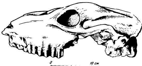
Рис. I. Иорибос из Квабеби (по А.К.Векуа, 1972)
