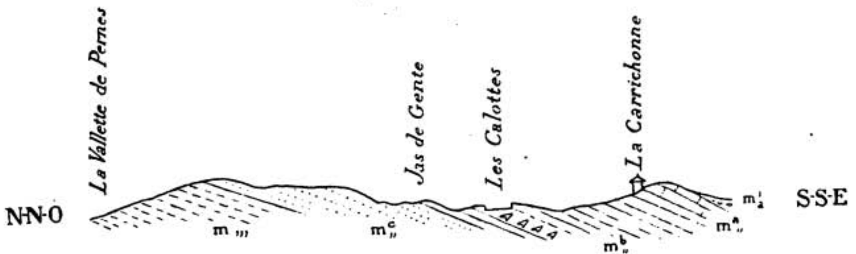
Fig. 1 : Coupe de l'Oligocène entre la Vallette de Pernes et la Carrichonne Mel. m'_{1} Burdig. inf.; m''^a marno-cal. à Helix cf. Ramondi ; m''^b marno-cal. à Lauræ ; m''^c sable à Ac. Filholi ; m''' Marnes vertes et Calc. de Pernes.
