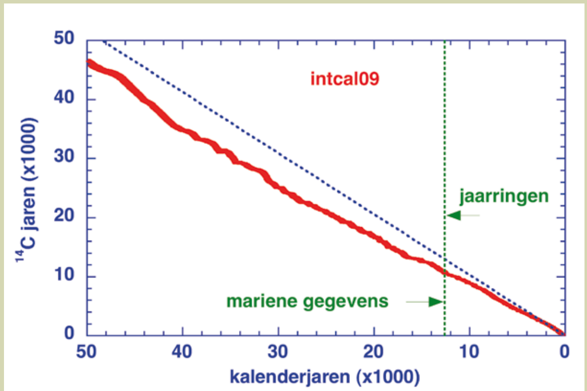
De ^{14}\text{C} -ijkgrafiek: het verband tussen ^{14}\text{C} dateringen in BP en de kalender tijdschaal, gebaseerd op dendrochronologie (tot 12.500 jaar geleden) en mariene gegevens.
