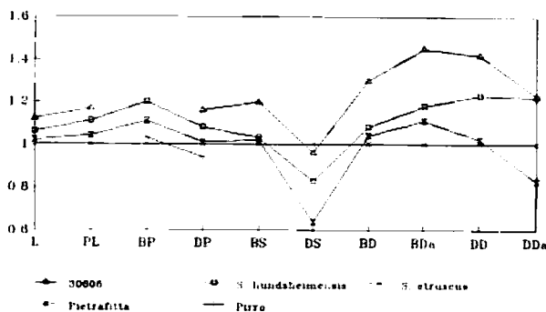
Fig. 3 - ratio diagram of the tibiae (standard S. etruscus ).
